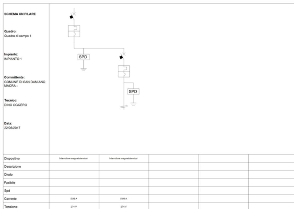
Fig. 9: Schema unifilare quadro "Quadro di campo 1"
