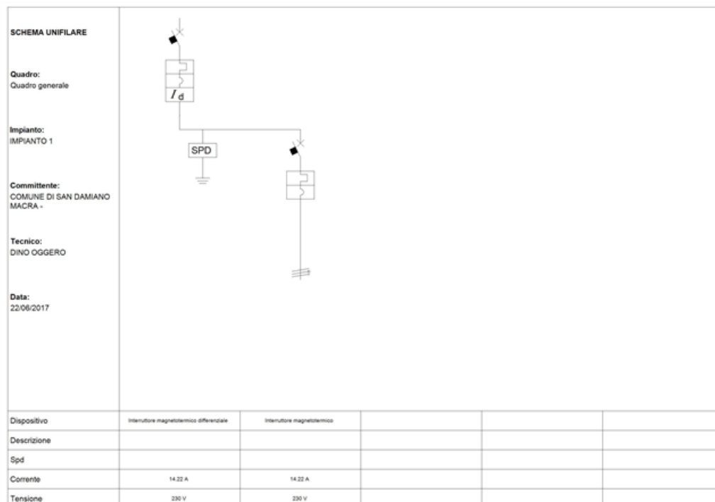
Fig. 6: Schema unifilare quadro "Quadro generale"
