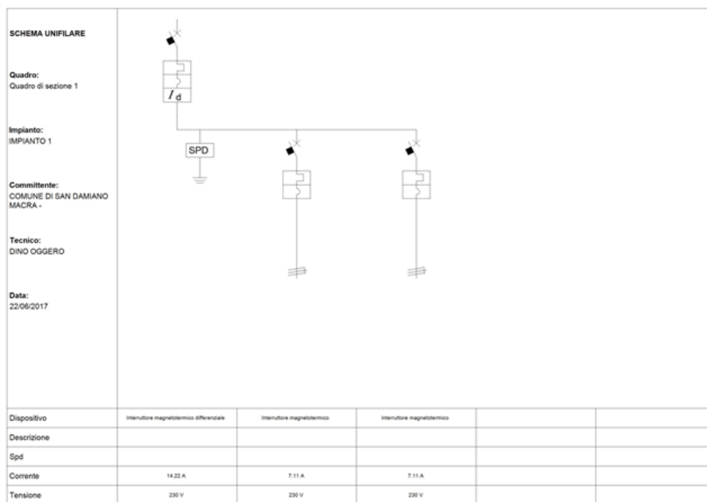
Fig. 8: Schema unifilare quadro "Quadro di sezione 1"
