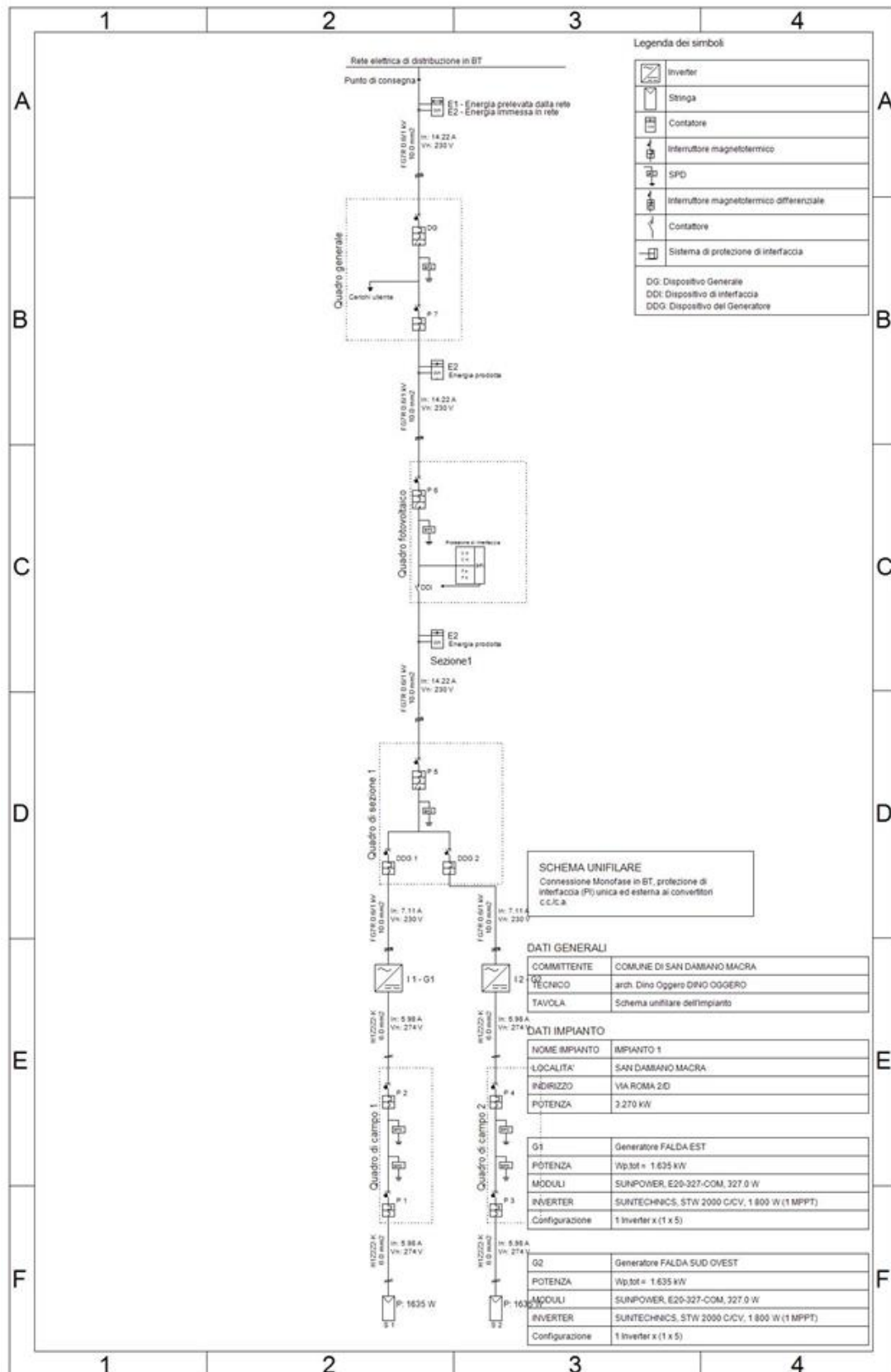
Fig. 11: Schema elettrico unifilare dell'impianto
