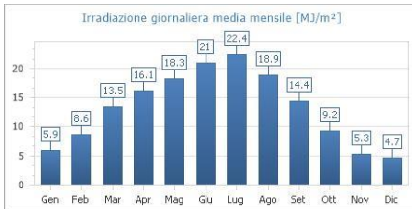
Fig. 1: Irradiazione giornaliera media mensile sul piano orizzontale [MJ/m 2 ]- Fonte dati: UNI 10349:2016 - Stazione di rilevazione: Boves
