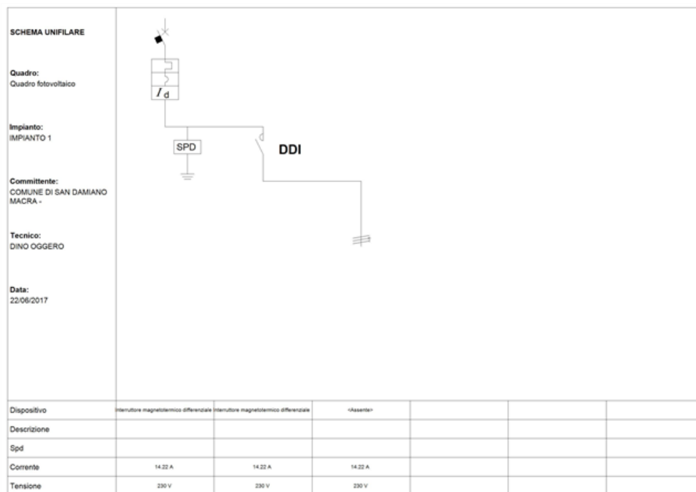
Fig. 7: Schema unifilare quadro "Quadro fotovoltaico"
