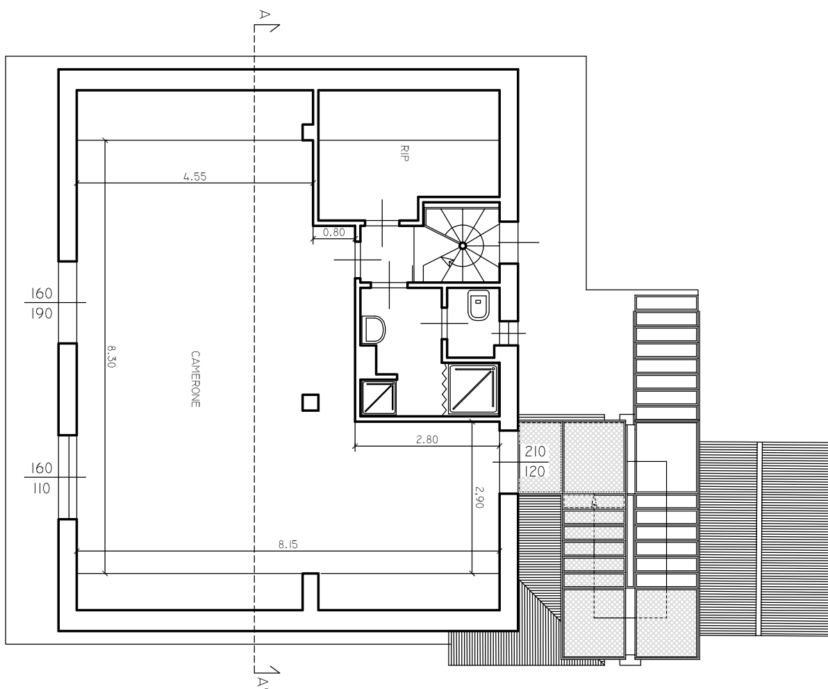
Piano sottotetto
