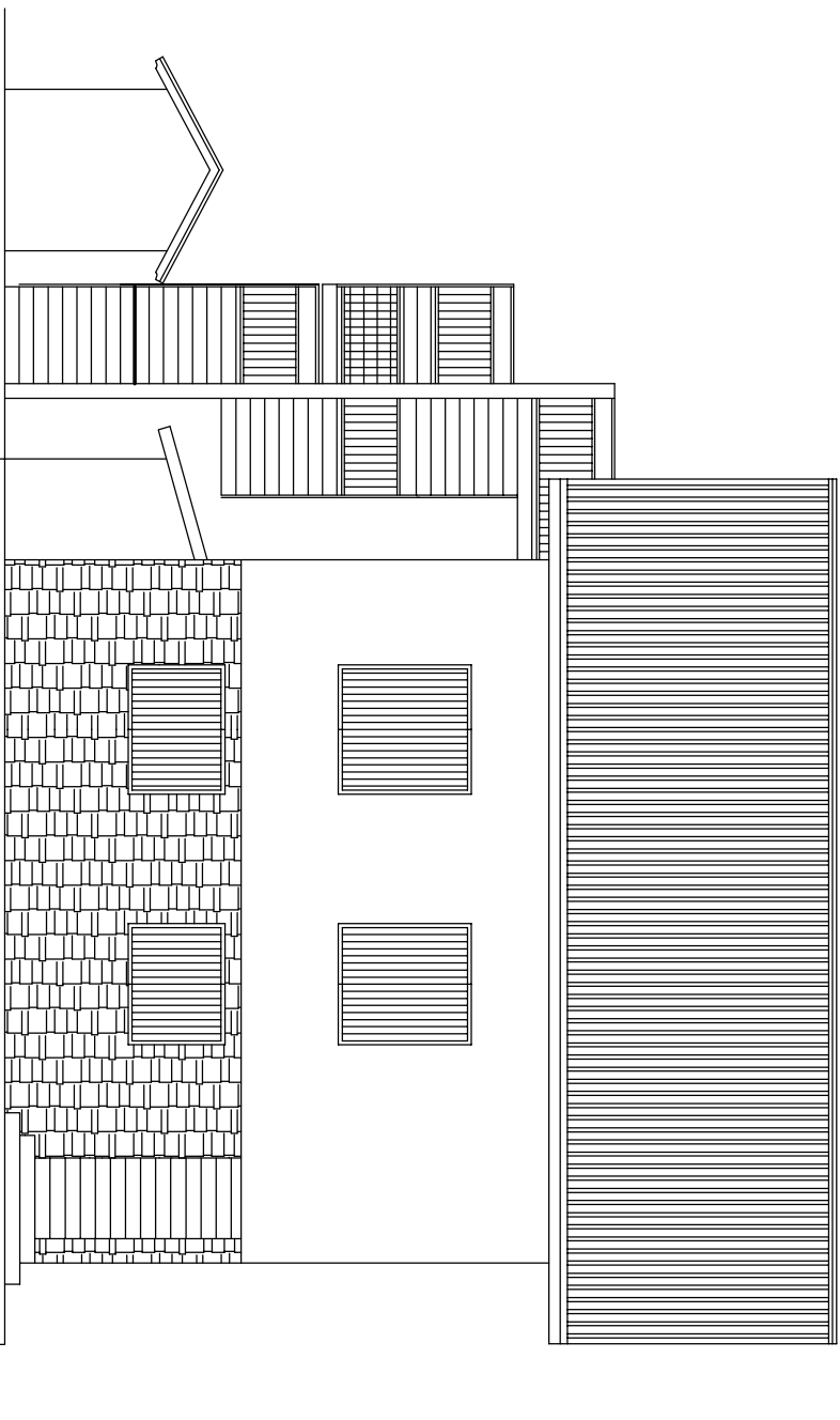
Prospetto nord
