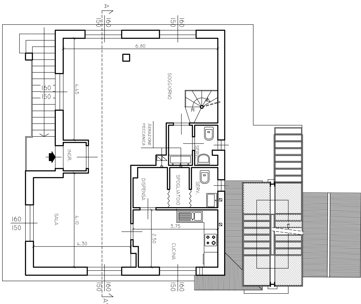
Piano primo
