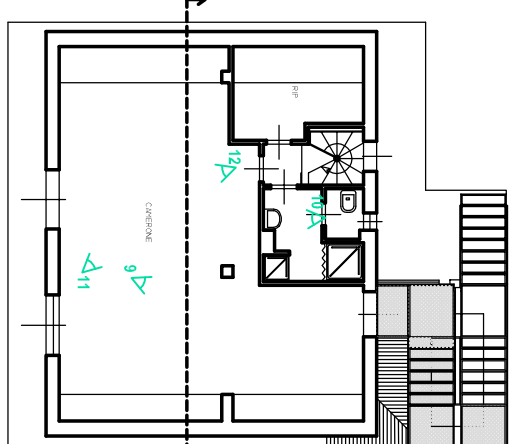
Piano sottotetto
